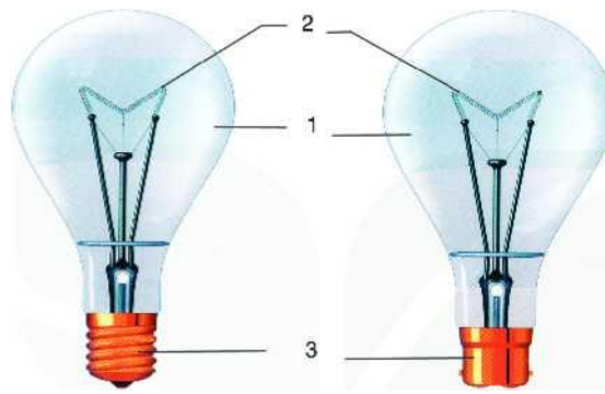
Cấu tạo của bóng đèn sợi đốt 1. Bóng thủy tinh 2. Sợi đốt 3. Đuôi đèn
